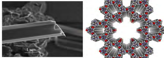
Tube creux hexagonal à paroi peptidique formé dans un cristal liquide. (Zhao, Dory)
